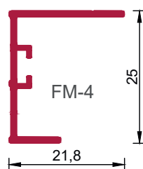
Seitenprofil FM-4 (Lagerlänge 450 cm) 3-000-255-X VE = 8 Stangen
