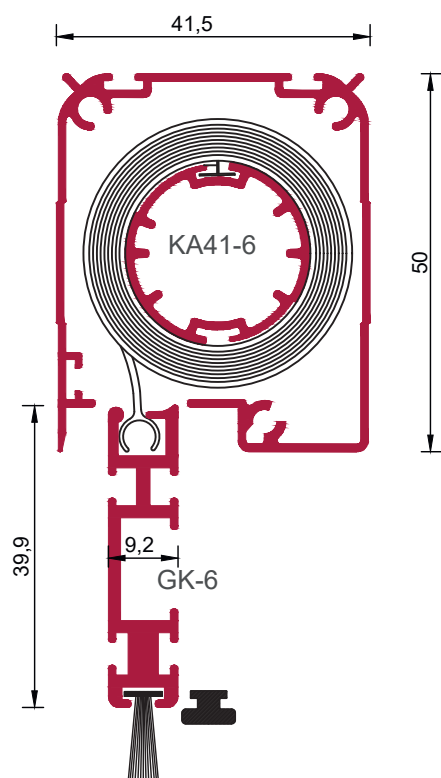
Klipsorollkassette KA41-6 3-000-100-X VE = 8 Stangen mit Gewebewelle
