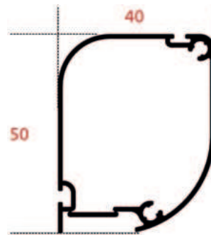
Abgerundeter Kasten
