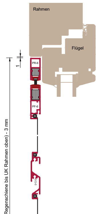
Vertikalschnitt PR1W und PR2W
