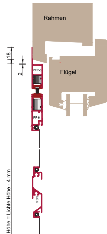
Vertikalschnitt PF1
