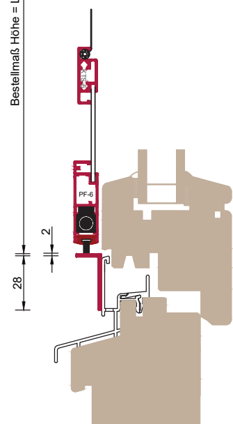
Vertikalschnitt PR1W und PR2W
