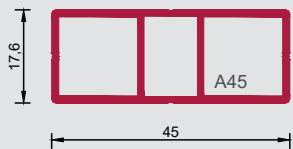
Montageprofil A-45 4-000-020-X
