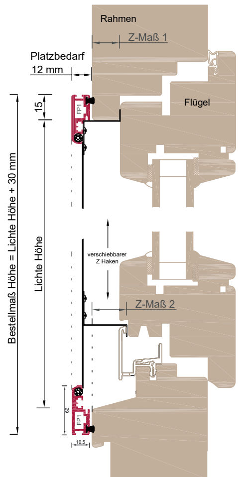
Vertikalschnitt FP1-3H
