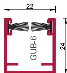
Bodenschiene GUB-6 3-000-260-X VE = 8 Stangen mit Bürste 4,8 x 10 cm
