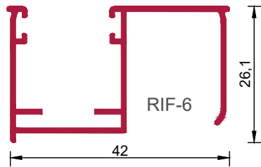
RIF-6 3-000-270-X U = 270 mm VE = 12 Stangen
