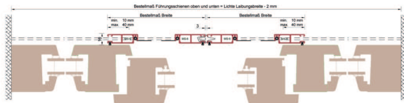
Variante MF-11-MS mit Bodenführung M2B und Winkelprofil W20-43
