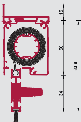
Frontmontage Linksroller mit Kassettenwinkel
