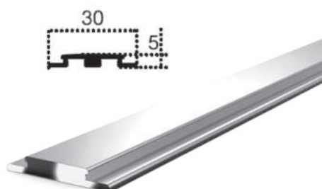
Optionale Schwelle
